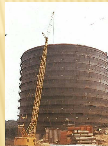
神根浄水場円盤型受水池（昭和46年）
